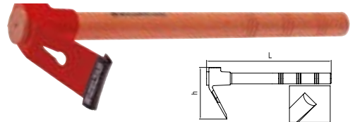
Özel alaşımlı çelik, İndüksiyonda sertleştirilmiş, Elektrostatik boyanmış, PVC ağız koruyucu Special steel, Induction hardened, Electrostatically painted, PVC cutting edge protector
